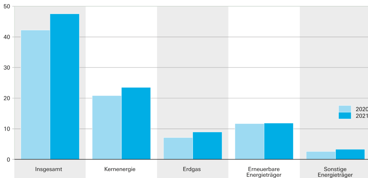
Abbildung 29: Bruttostromerzeugung in Kraftwerken der allgemeinen Versorgung in Bayern 2020 und 2021 nach Energieträgern in Terawattstunden
